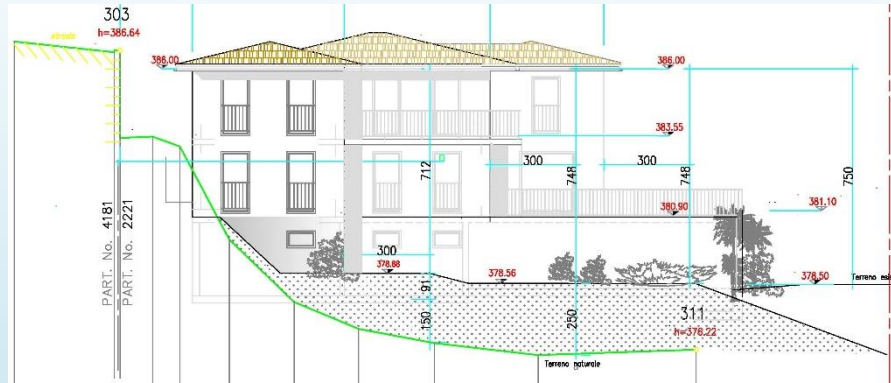
Facciata
