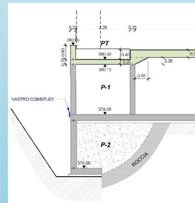
Sezione
