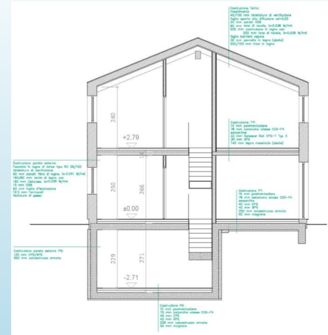
Sezione
